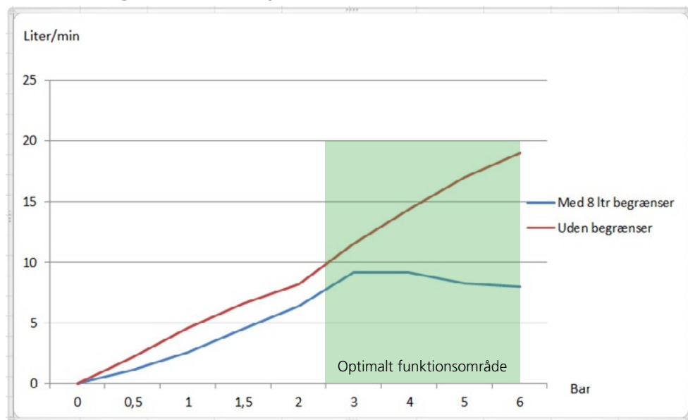
Vandforbrug i forhold til tryk
